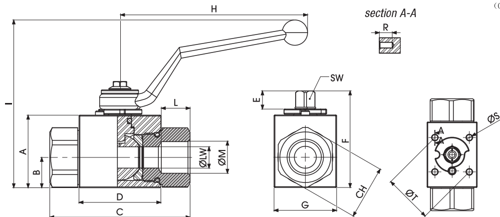
英制直管螺纹 (G螺纹)
