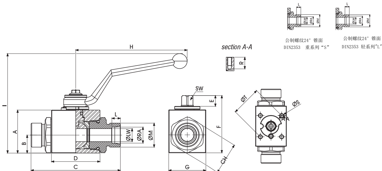
公制螺纹24° 锥面DIN2353重系列（S）球体尺寸及工作压力
